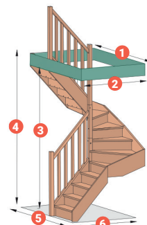
Configuratie 5: Dubbele kwart links
