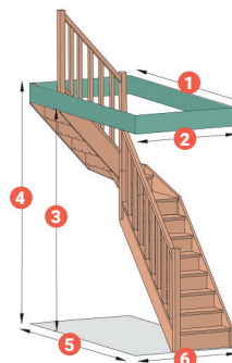
Configuratie 4: Middenkwart links
