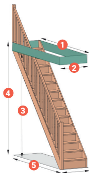
Configuratie 1: Rechte trap
