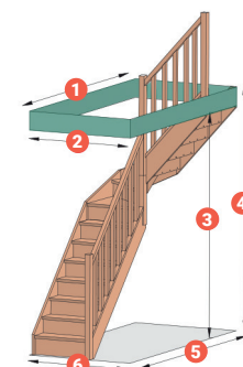
Configuratie 9: Middenkwart rechts
