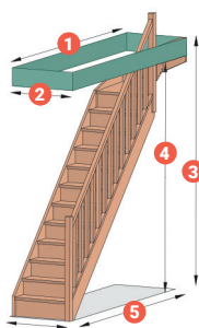
Configuratie 8: Bovenkwart rechts
